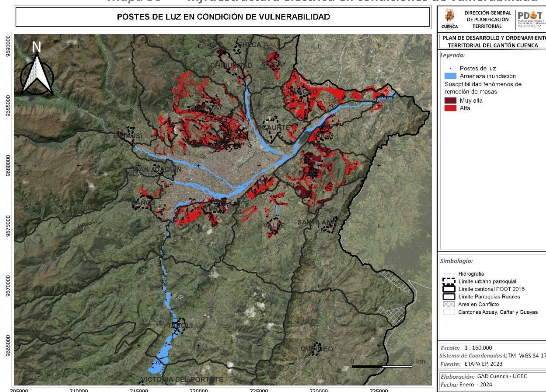
Mapa 56 Infraestructura eléctrica en condiciones de vulnerabilidad
