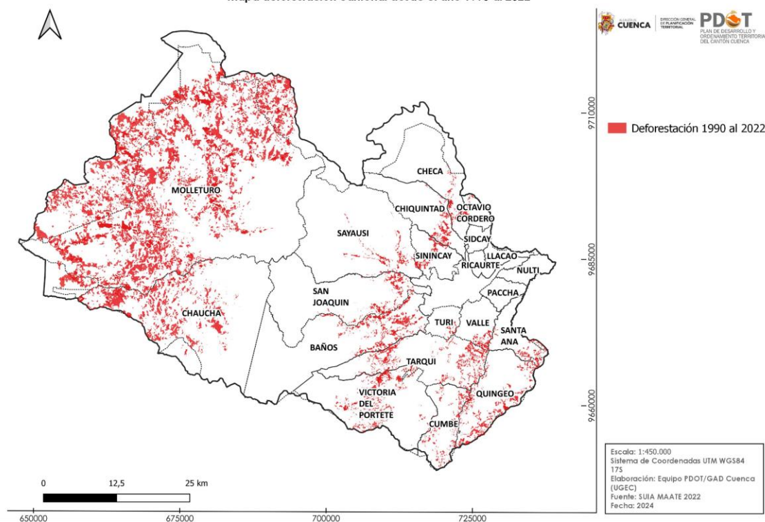
Mapa 32 Deforestación cantonal desde el año 1990 al 2022
