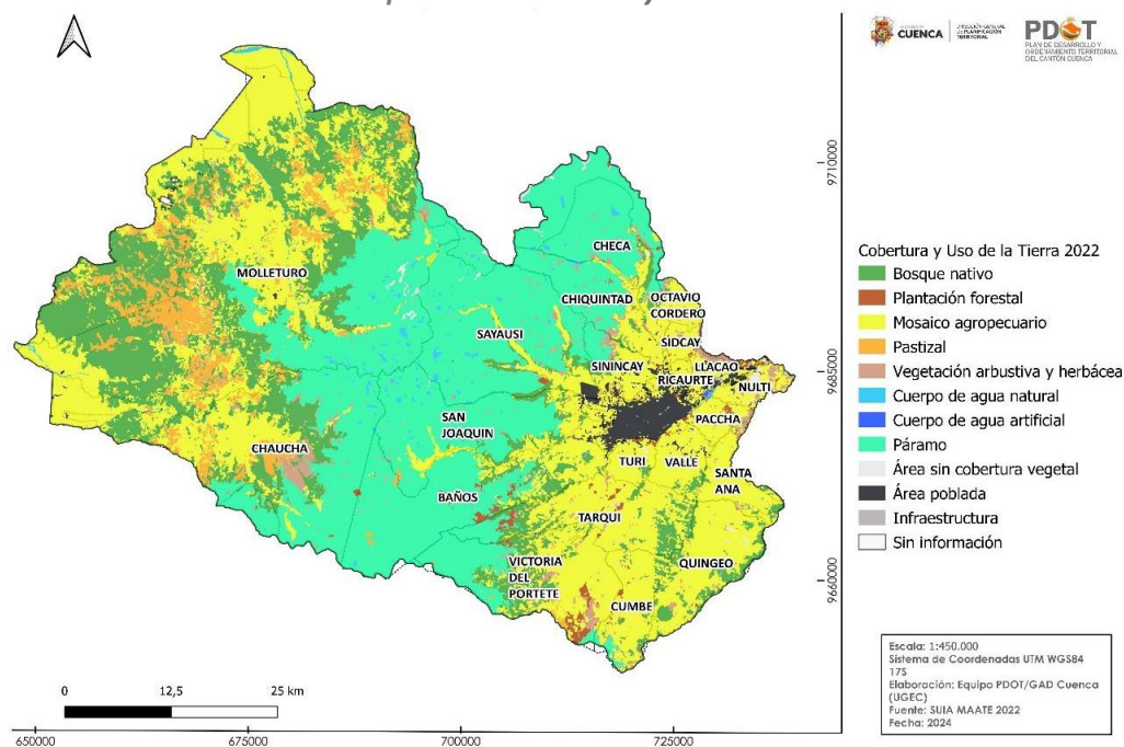
Mapa 9 Cobertura y uso de la tierra MAATE 2022
