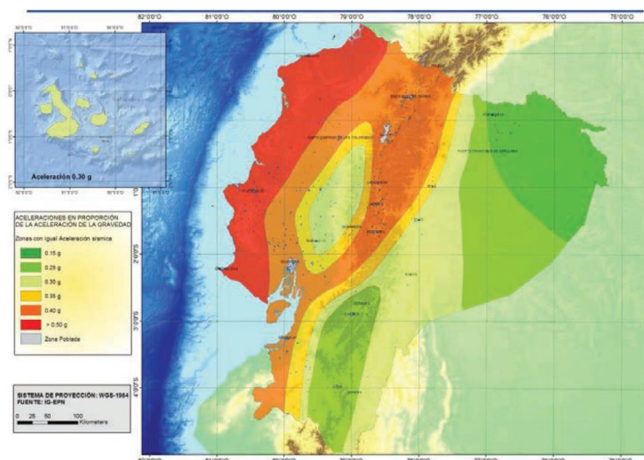
Mapa 16 Ecuador, zonas sísmicas para propósitos de diseño y valor del factor de zona
