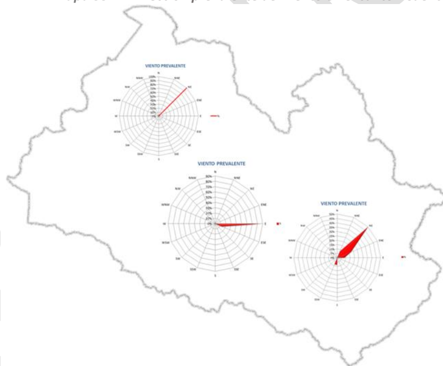
Mapa 33 Dirección prevalente del viento en el cantón Cuenca
