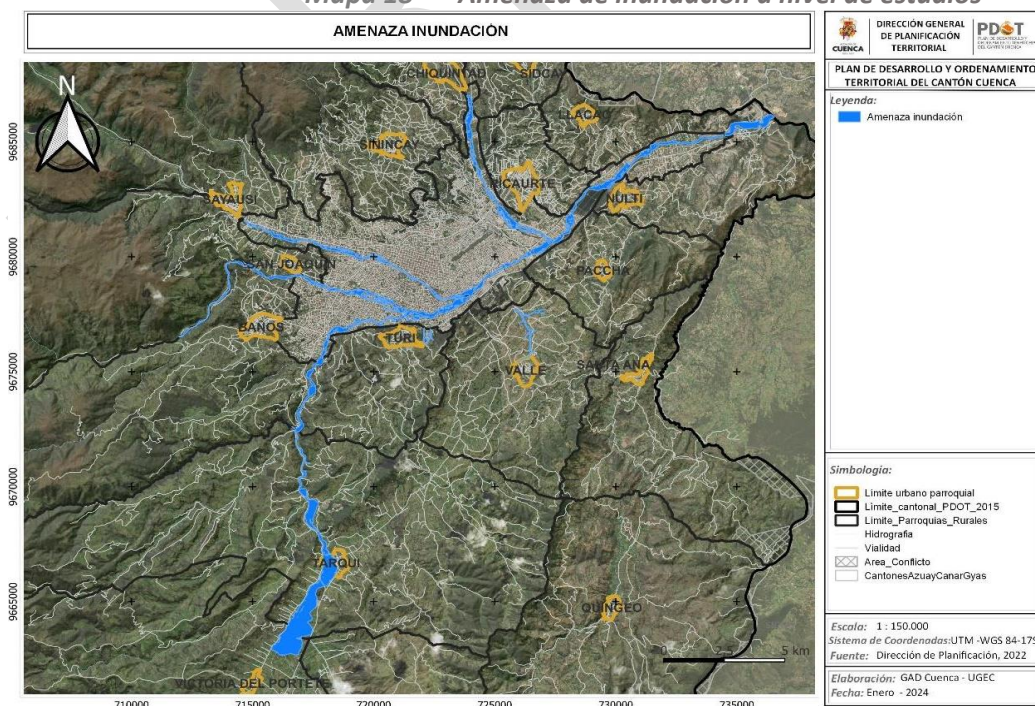
Mapa 18 Amenaza de inundación a nivel de estudios
