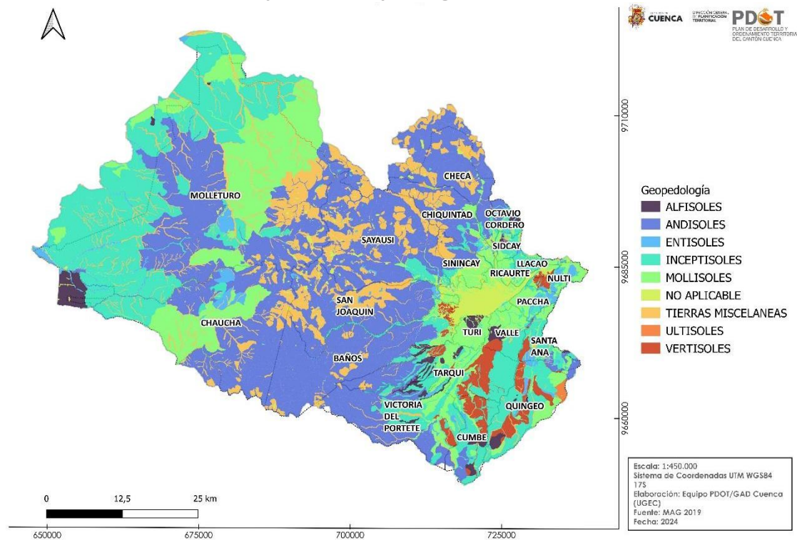
Mapa 10 Geopedología del suelo - taxonomía
