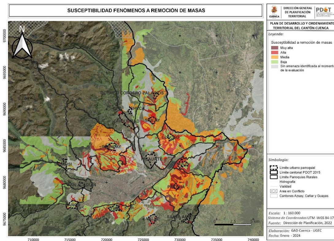
Mapa 12 Susceptibilidad a fenómenos de remoción de masas a mayor detalle
