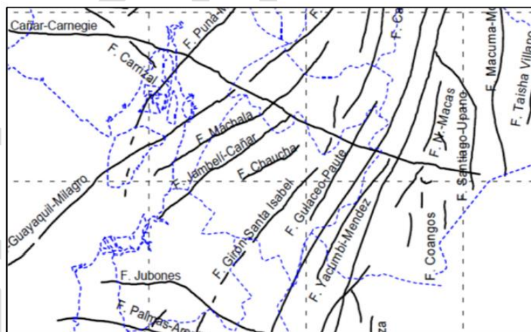
Mapa 15 Fallas ubicadas en el Austro del Ecuador Ubicación Proyectos EMUVI
