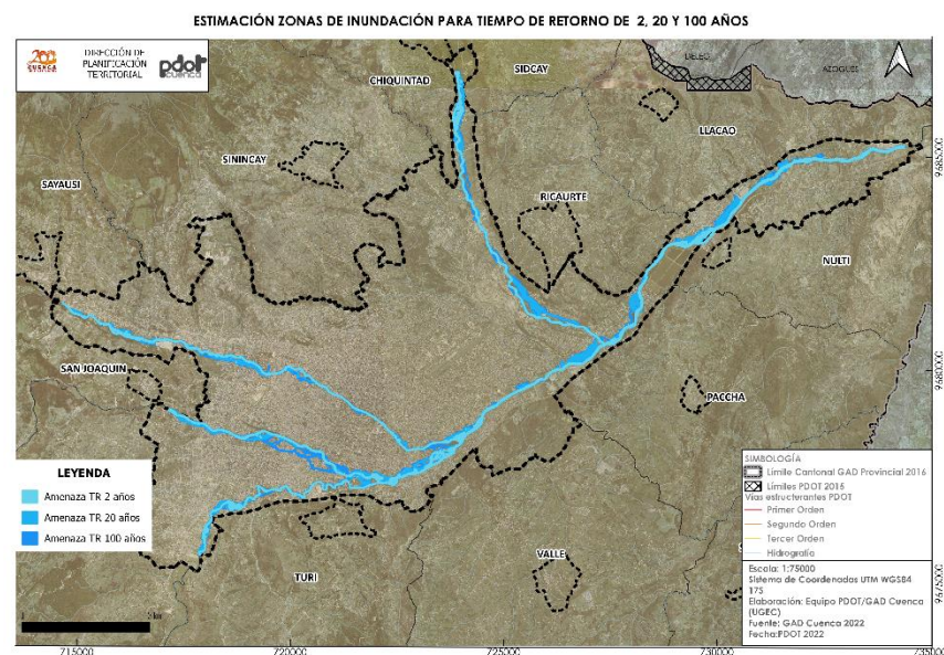
Mapa 22. Estimación zonas de inundación TR 2, 20 y 100 años
