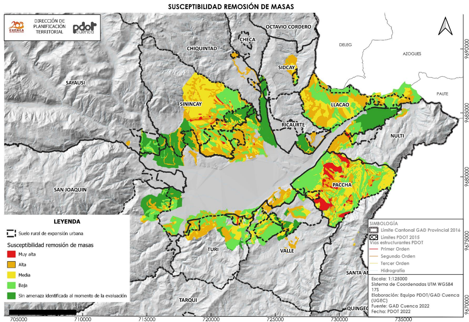
Mapa 21. Zonas con susceptibilidad a remoción de masas
