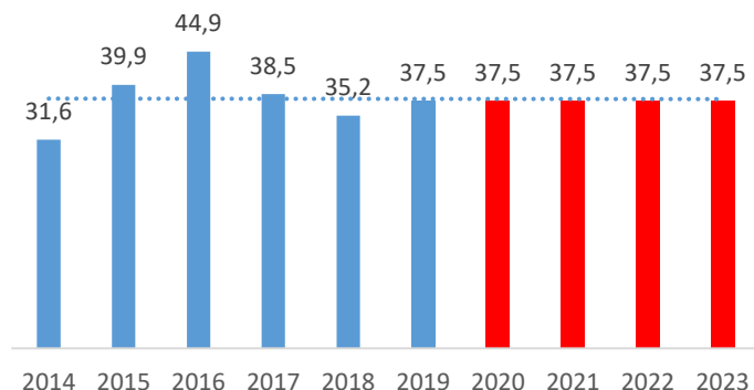
Figura 11. Promedio anual de material particulado PM10.
