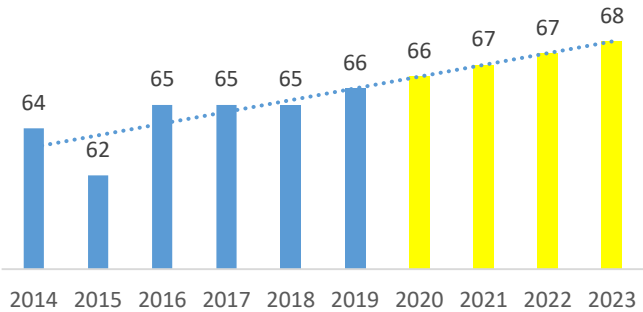
Figura 13. Índice de calidad del Agua WQI Ucubamba.
