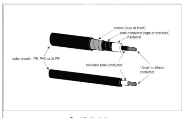
Figura 14-2. cable primario
