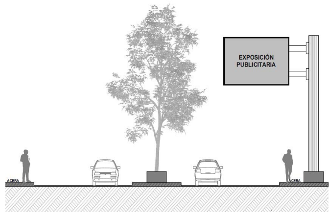
Figura 5. Tipo D: Voladizo - Publicidad o propaganda exterior en acera
