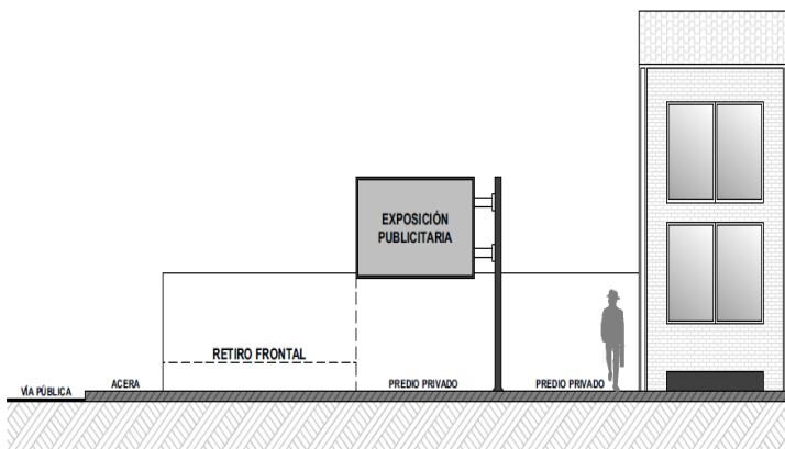
Figura. 19.- Tipo D - En Voladizo en predios edificados o en proceso de edificación.
