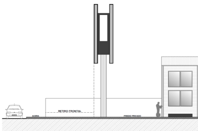
Figura 17.- Tipo A - Publicidad o propaganda Exterior: Alta en predios privados, edificados o en proceso de edificación.- Área de exposición paralela al eje de la vía.
