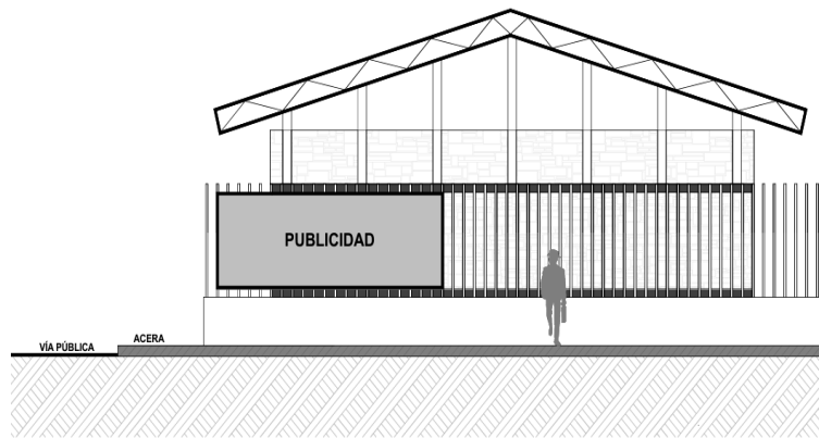
Figura 14. Tipo L - Lona.- Publicidad o propaganda exterior Lona en cerramiento o fachada.
