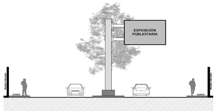
Figura 4. Tipo D: Voladizo - Publicidad o propaganda exterior en medianas o bandas centrales (parterres)
